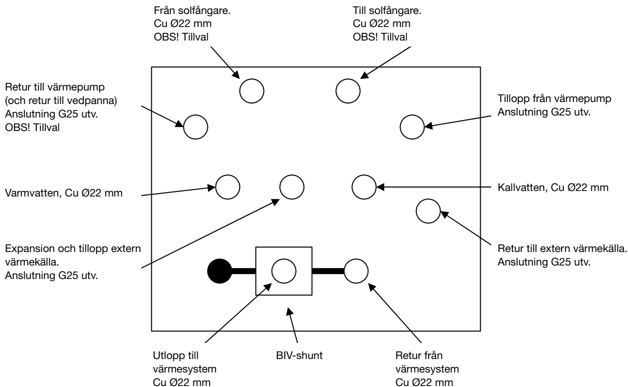
Akkumulatortankens framsida
