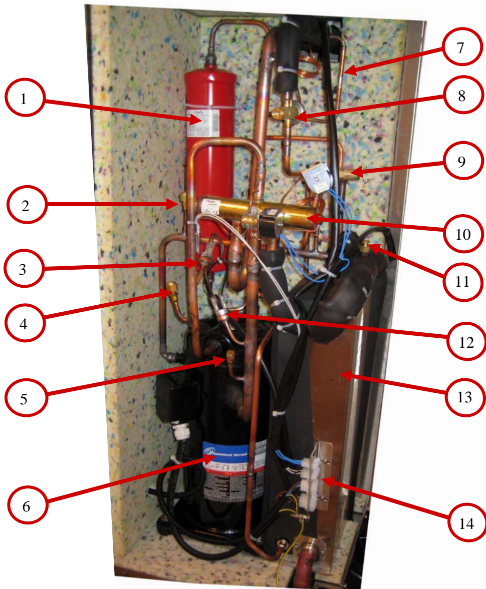
Figur 2. Komponentplacering Polaris.
