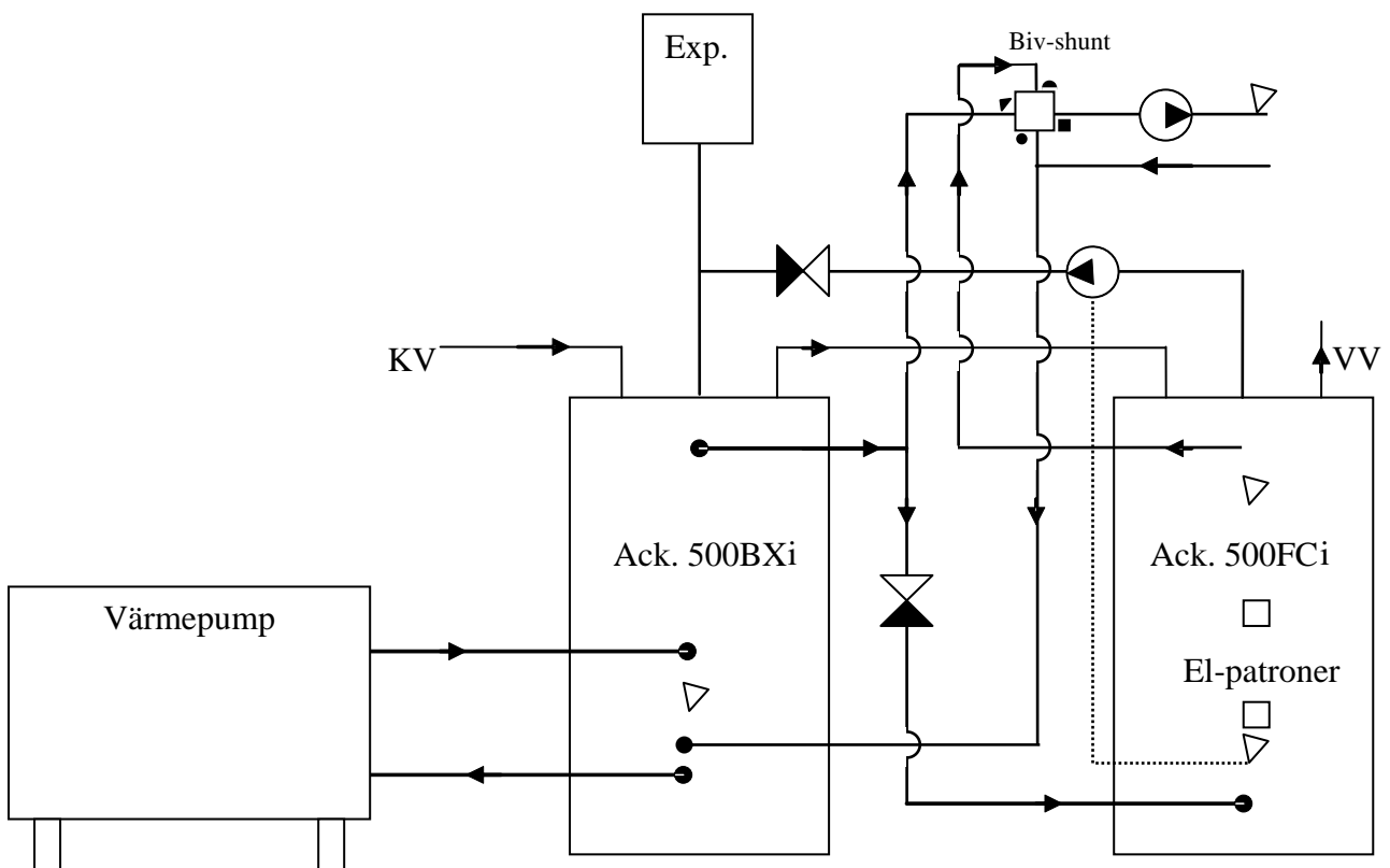
Figur 7 Tvåtanksystem
