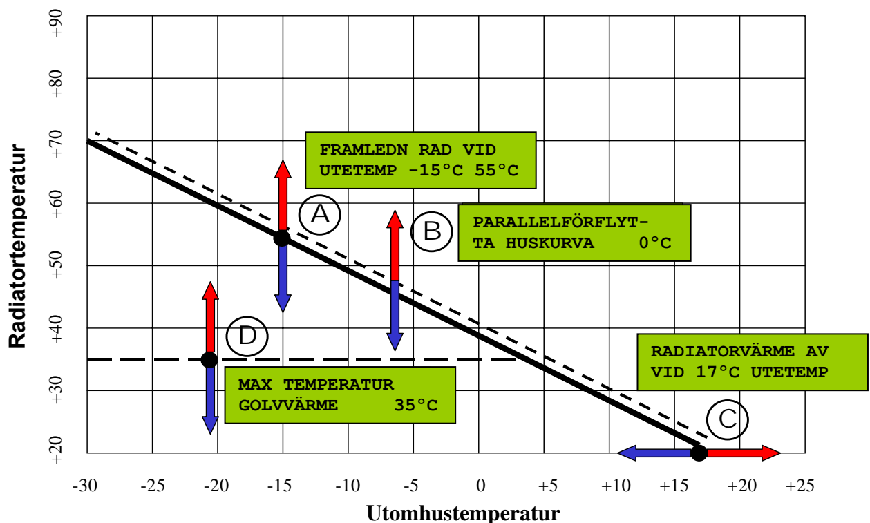
Figur 20. Huskurva
