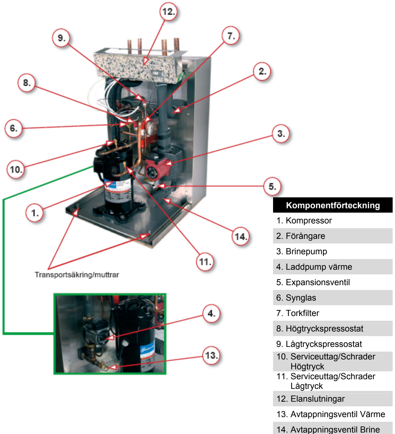
Figur 8. Komponentplacering Exotic
