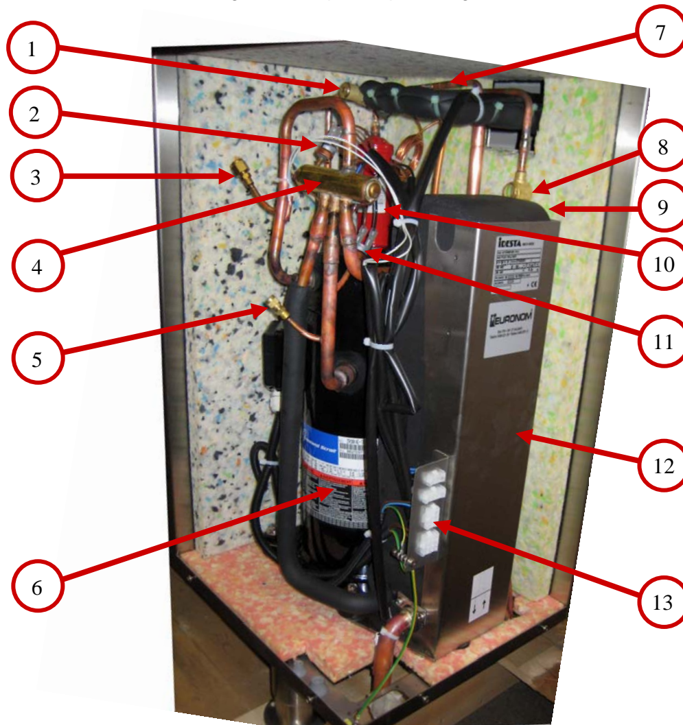
Figur 1. Komponentplacering ExoAir
