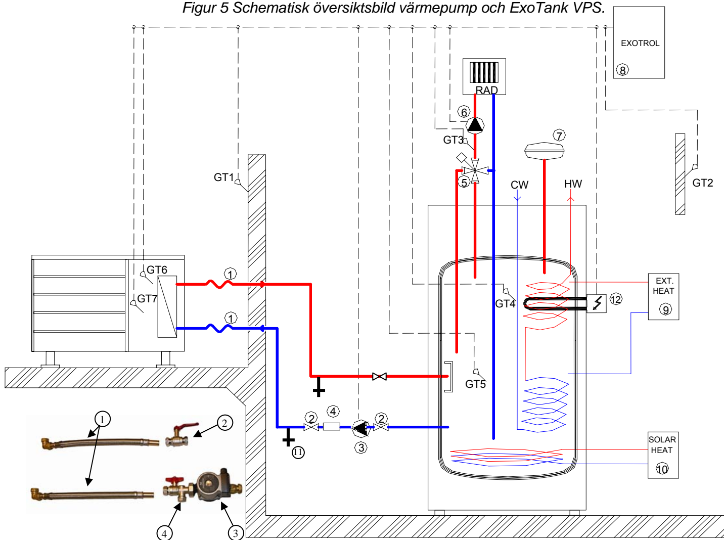
Figur 5 Schematisk översiktsbild värmepump och ExoTank VPS.
